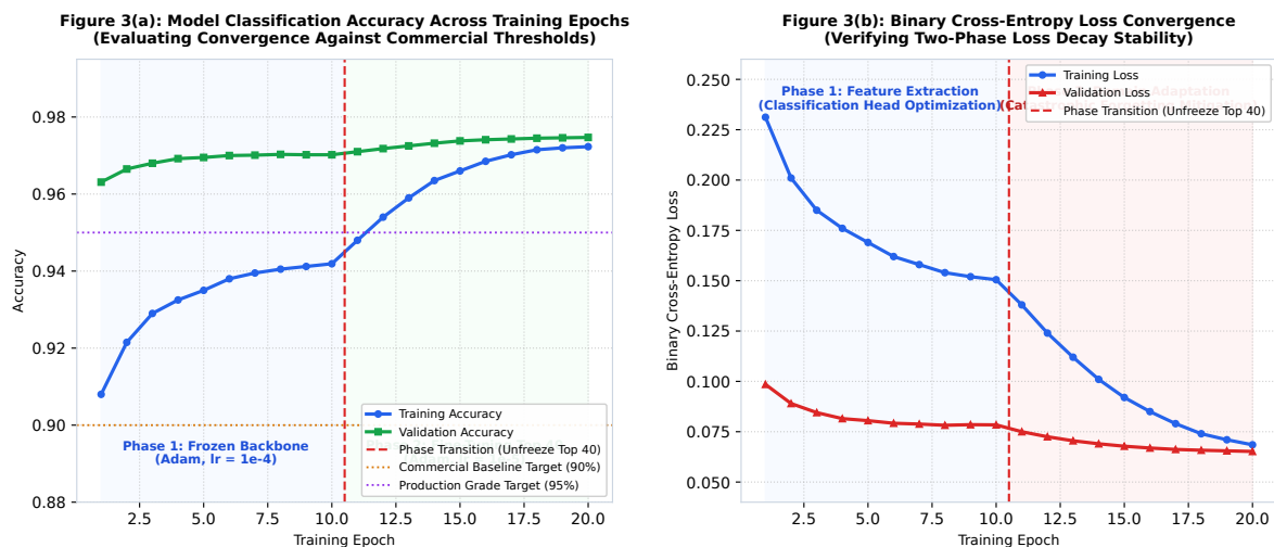
รูปที่ 3: เส้นทางการเรียนรู้ 2 ขั้นตอนของโมเดล MobileNetV2: (a) ความแม่นยำ (Accuracy) เทียบกับเกณฑ์เป้าหมาย 90% และ 95% (b) ค่าความสูญเสีย (Binary Cross-Entropy Loss)
